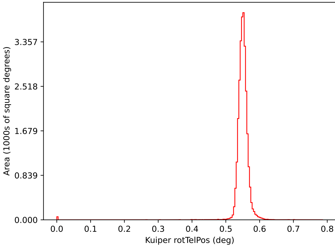
too_elab_r16_d2_griz_v3.4_10yrs i: Kuiper rotTelPos
