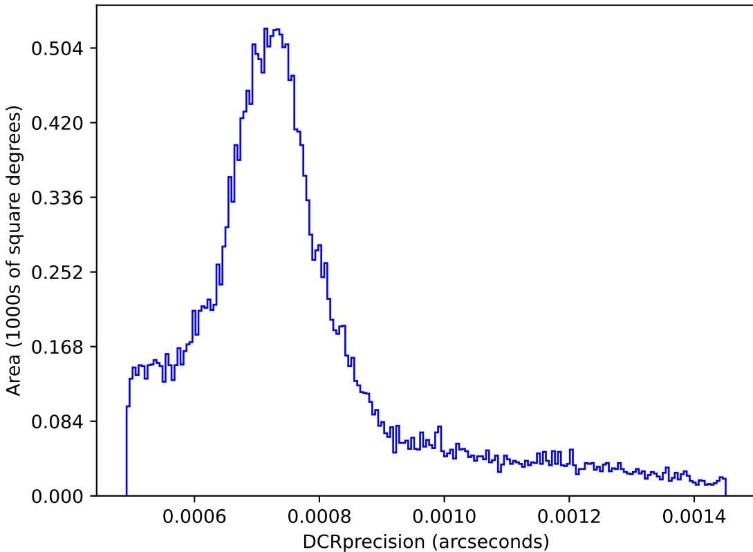
too_elab_r16_d2_griz_v3.4_10yrs : DCRprecision
