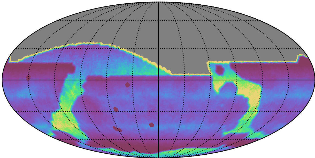
too_elab_r16_d2_giz_v3.4_10yrs : DCRprecision
