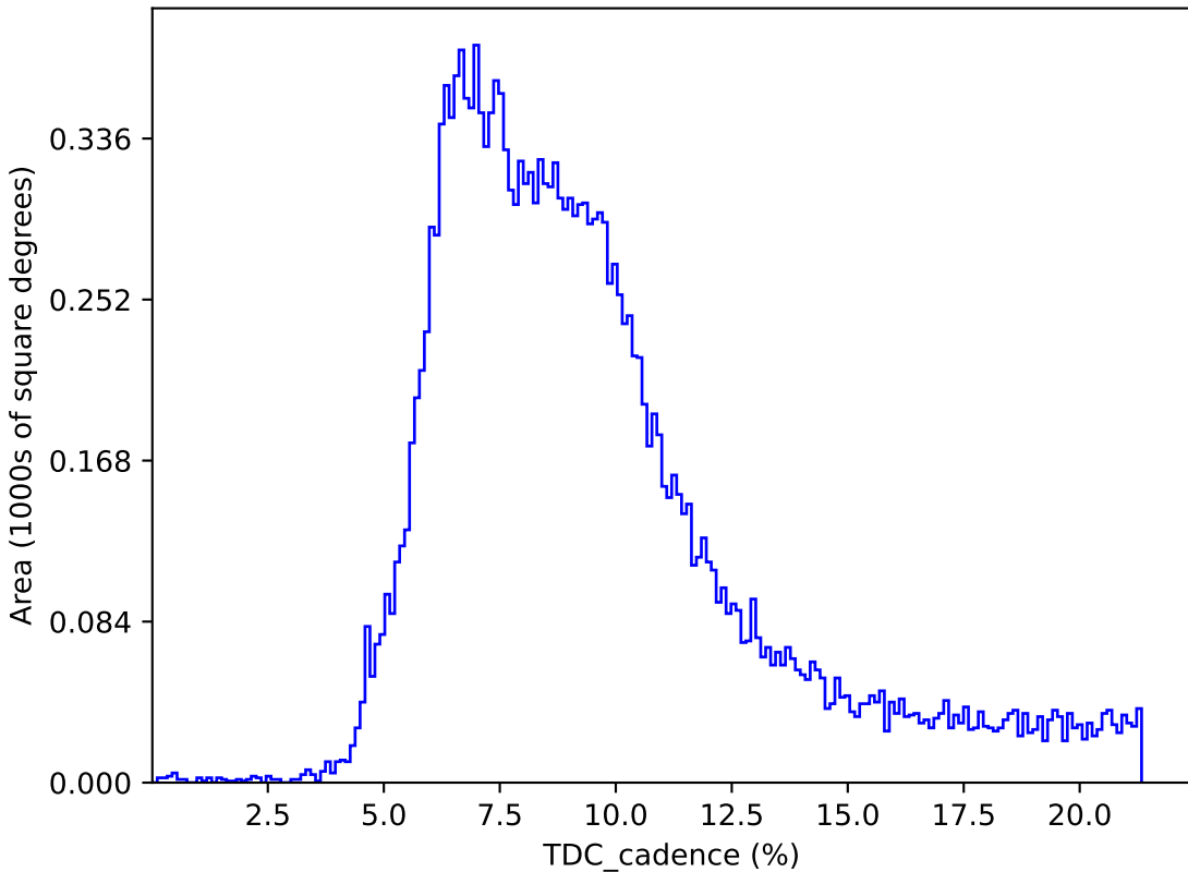
too_elab_r128_d3_ugrizy_v3.4_10yrs : TDC_cadence
