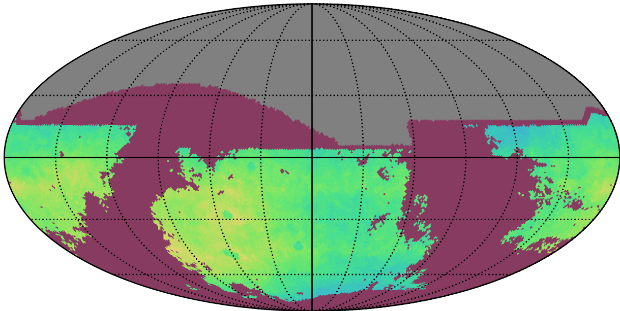
too_elab_r128_d3_ugrizy_v3.4_10yrs i: NgalScale
