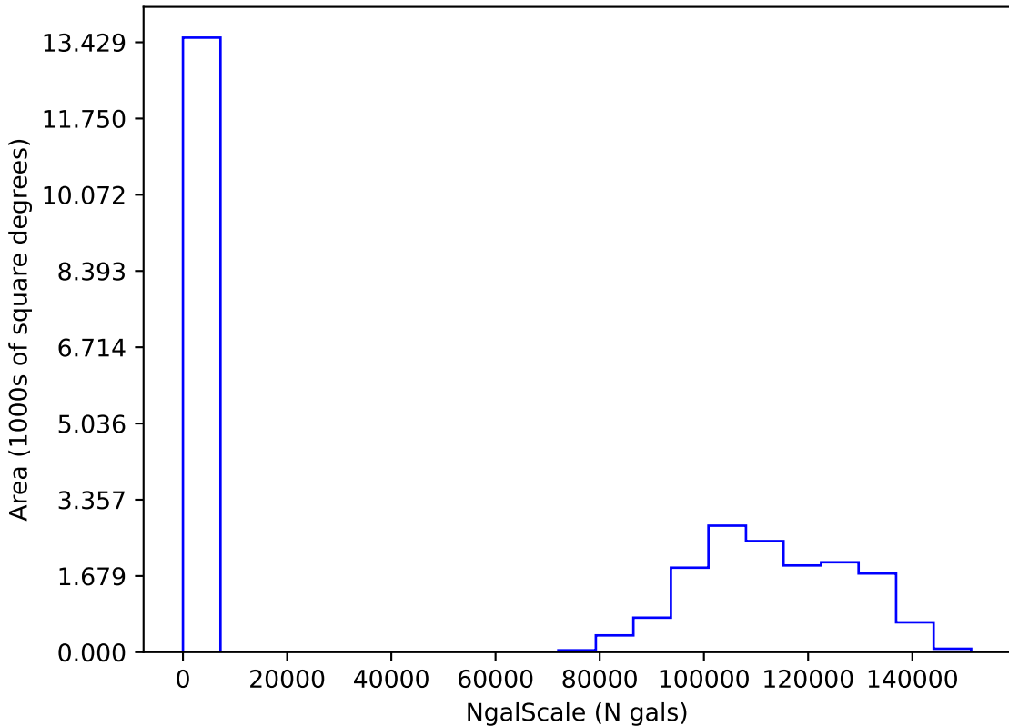
too_elab_r128_d3_ugrizy_v3.4_10yrs i: NgalScale
