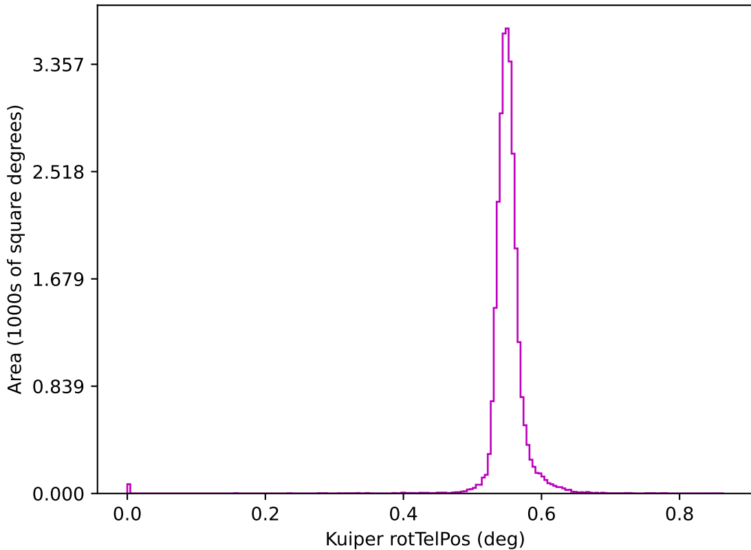
too_elab_r128_d3_ugrizy_v3.4_10yrs z: Kuiper rotTelPos
