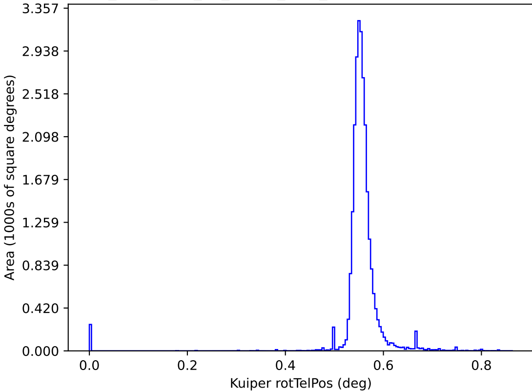
too_elab_r128_d3_ugrizy_v3.4_10yrs y: Kuiper rotTelPos
