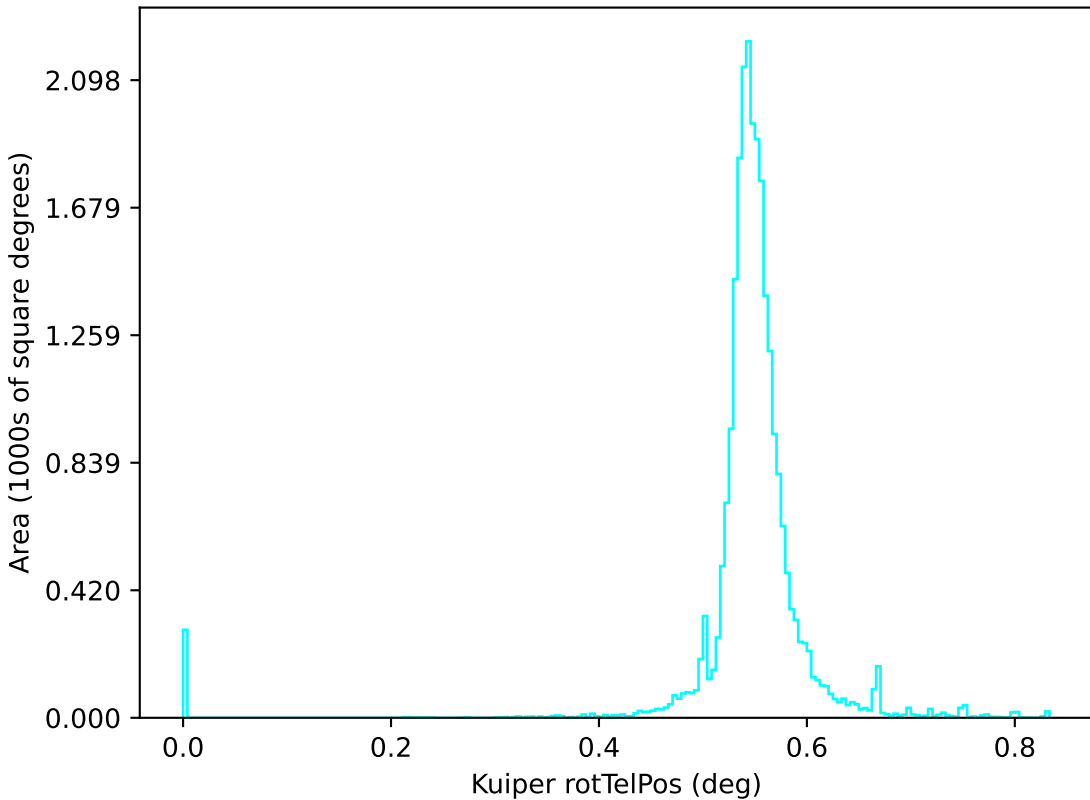
too_elab_r128_d3_ugrizy_v3.4_10yrs u: Kuiper rotTelPos
