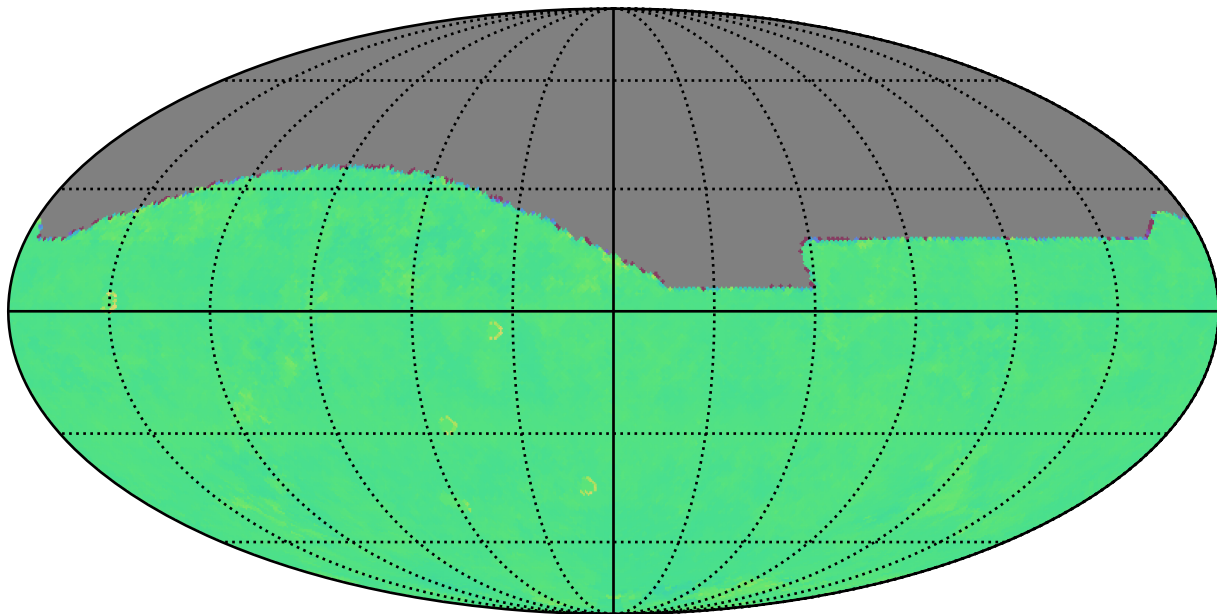
too_elab_r128_d3_ugrizy_v3.4_10yrs i: Kuiper rotTelPos
