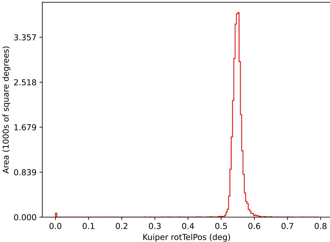
too_elab_r128_d3_ugrizy_v3.4_10yrs i: Kuiper rotTelPos
