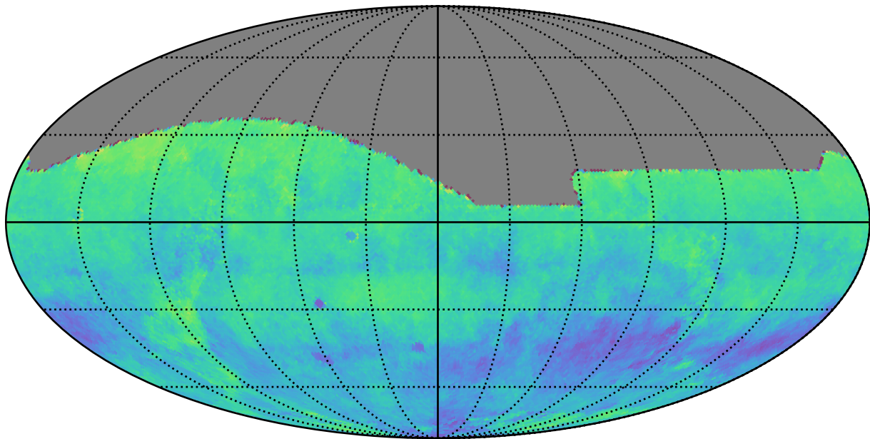
too_elab_r128_d3_ugrizy_v3.4_10yrs i: Kuiper rotSkyPos
