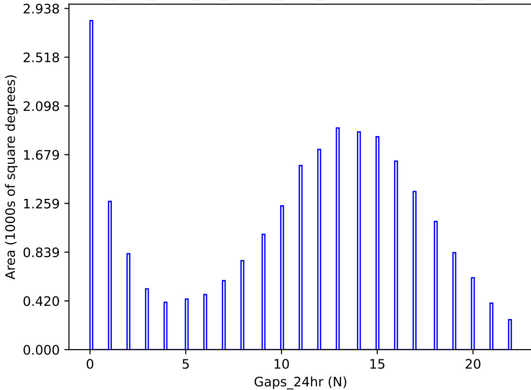
too_elab_r128_d3_ugrizy_v3.4_10yrs y band: Gaps_24hr
