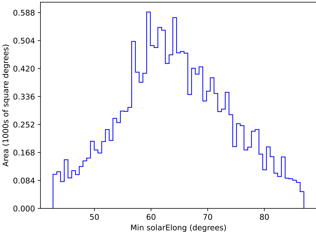
too_elab_r128_d3_ugrizy_v3.4_10yrs WFD y band: Min solarElong
