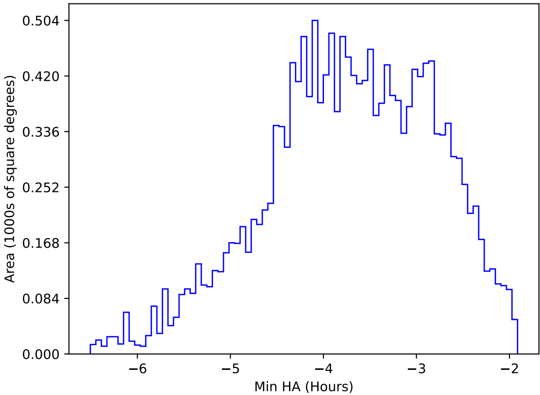
too_elab_r128_d3_ugrizy_v3.4_10yrs WFD y band: Min HA
