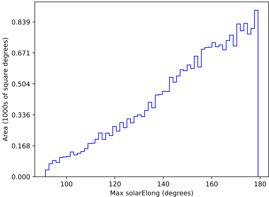
too_elab_r128_d3_ugrizy_v3.4_10yrs All sky y band: Max solarElong
