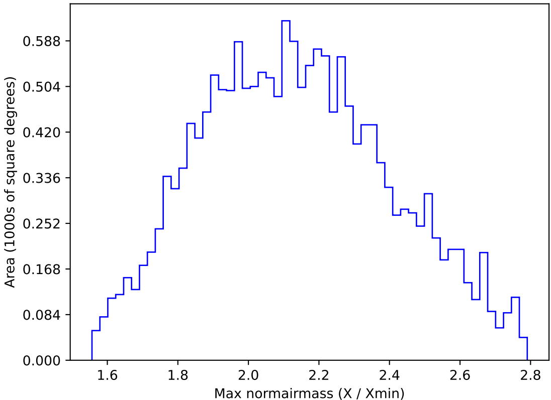
too_elab_r128_d3_ugrizy_v3.4_10yrs WFD y band: Max normairmass
