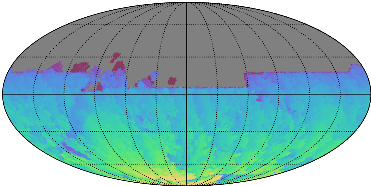
too_elab_r128_d3_ugrizy_v3.4_10yrs All sky y band: Max HA
