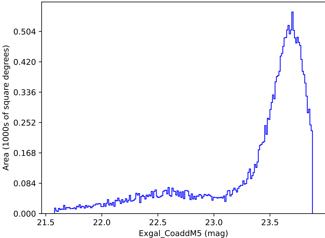
too_elab_r128_d3_ugrizy_v3.4_10yrs Yr 1 y band: Exgal_CoaddM5
