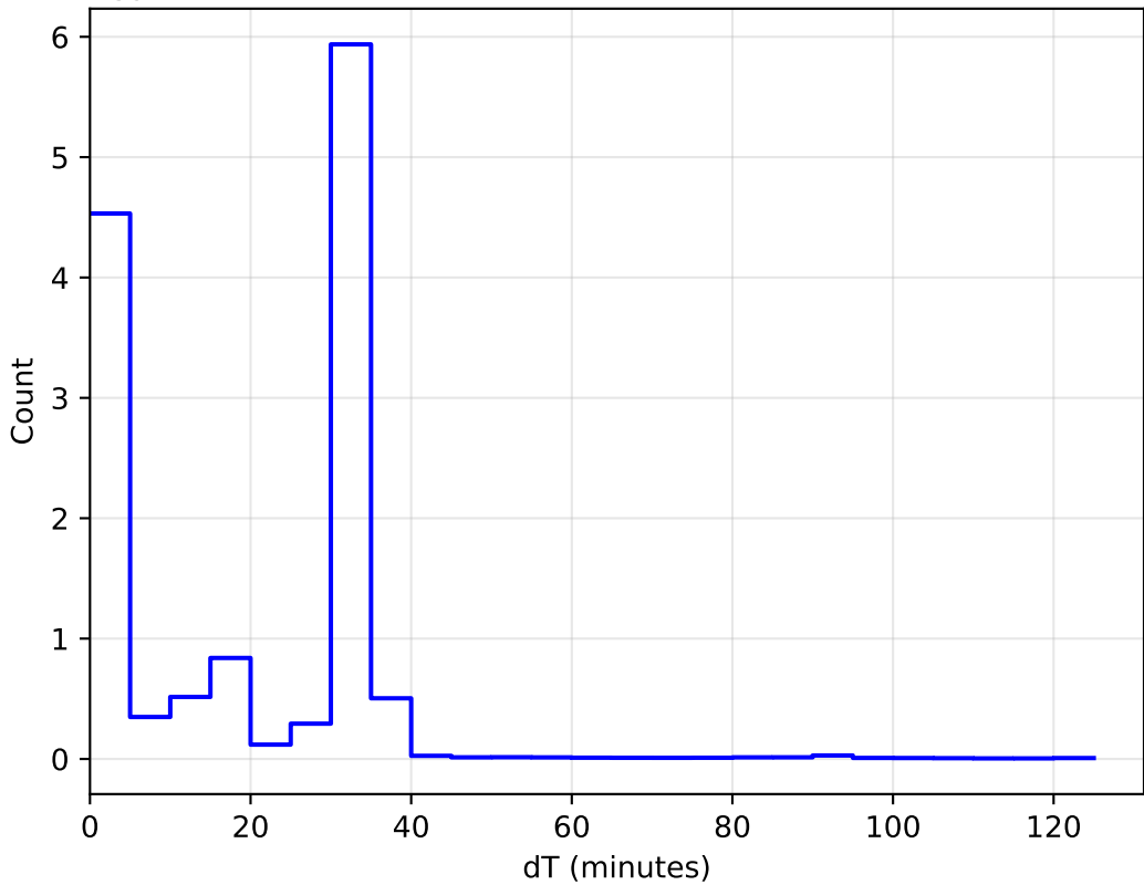
too_elab_r128_d3_ugrizy_v3.4_10yrs All sky: DeltaT Histogram 1e6
