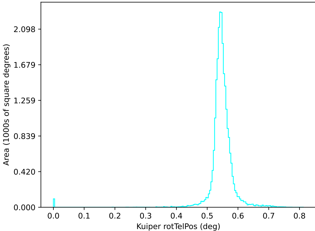
too_elab_r128_d3_gz_v3.4_10yrs u: Kuiper rotTelPos
