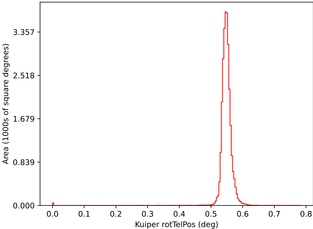
too_elab_r128_d3_gz_v3.4_10yrs i: Kuiper rotTelPos
