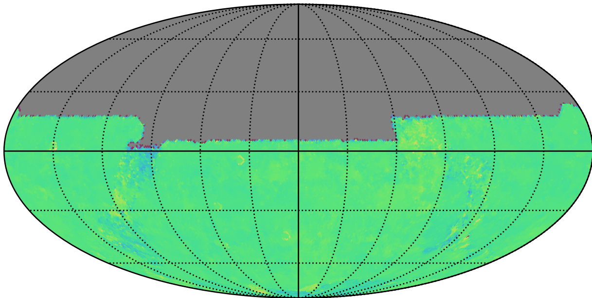
too_elab_r128_d3_griz_v3.4_10yrs u: Kuiper rotTelPos
