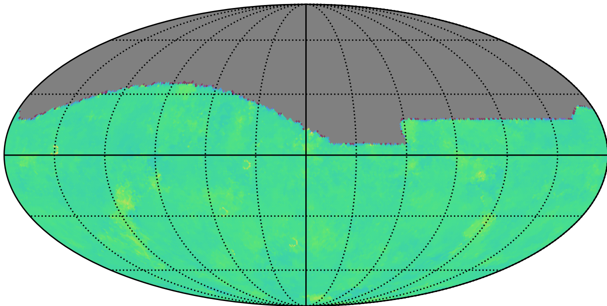
too_elab_r128_d3_griz_v3.4_10yrs g: Kuiper rotTelPos
