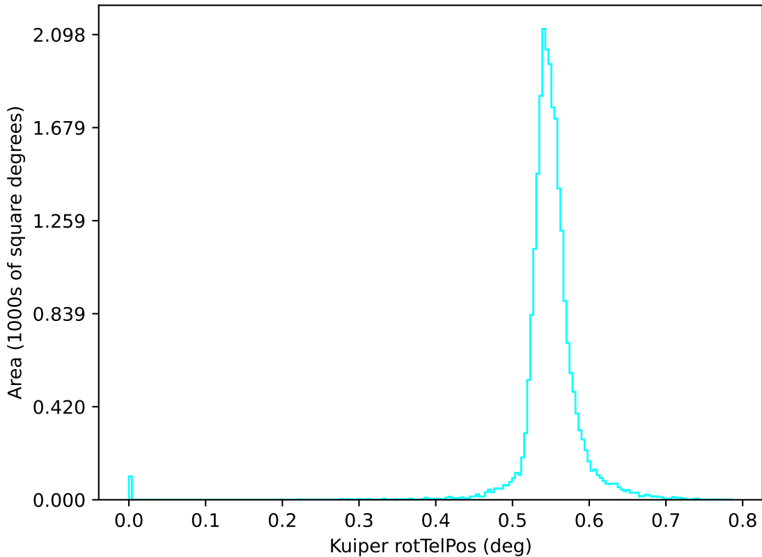
too_elab_r128_d3_giz_v3.4_10yrs u: Kuiper rotTelPos
