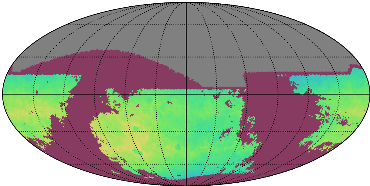
too_elab_r128_d2_ugrizy_v3.4_10yrs i: NgalScale
