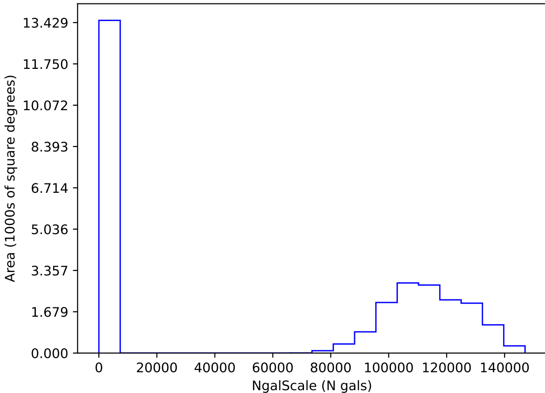
too_elab_r128_d2_ugrizy_v3.4_10yrs i: NgalScale
