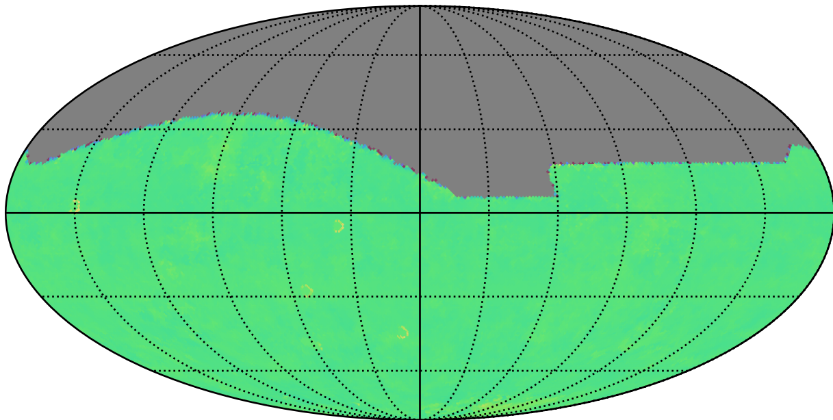
too_elab_r128_d2_ugrizy_v3.4_10yrs i: Kuiper rotTelPos
