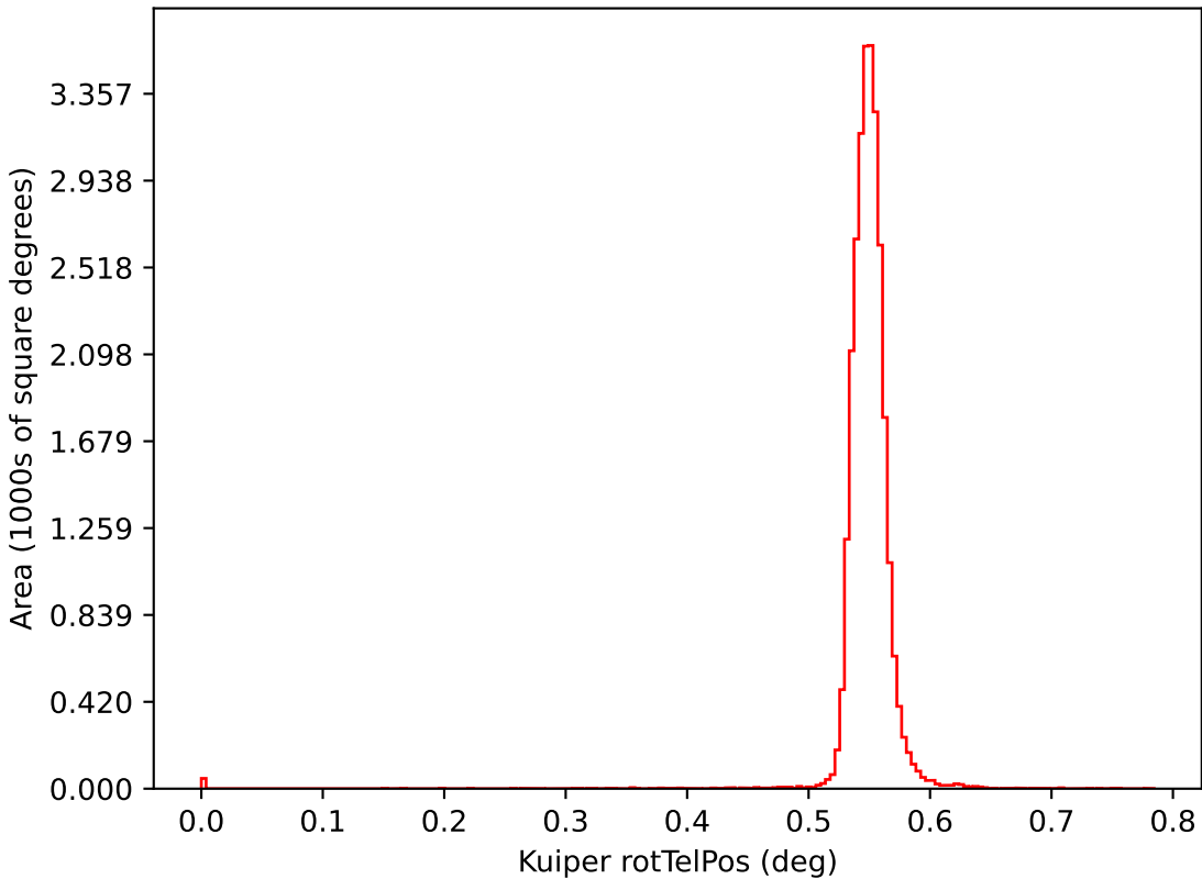
too_elab_r128_d2_ugrizy_v3.4_10yrs i: Kuiper rotTelPos
