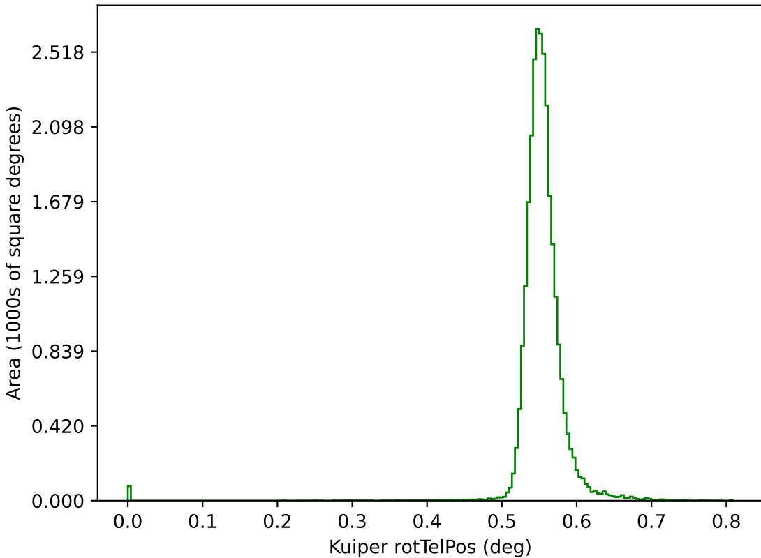
too_elab_r128_d2_ugrizy_v3.4_10yrs g: Kuiper rotTelPos
