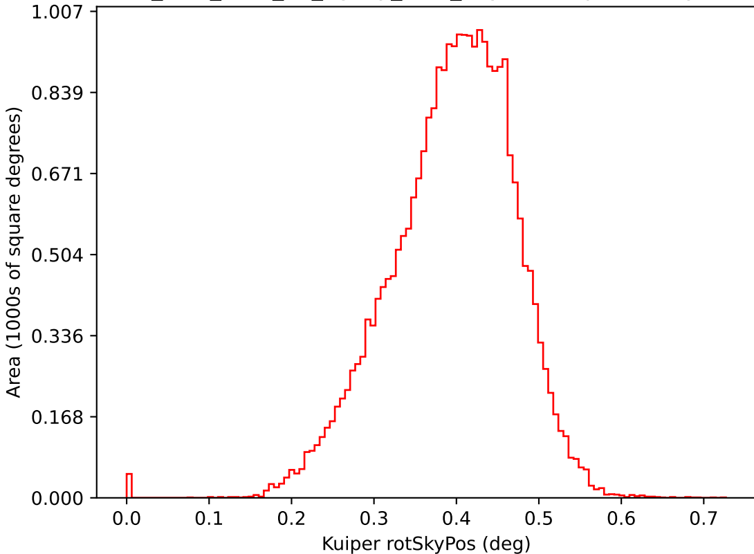
too_elab_r128_d2_ugrizy_v3.4_10yrs i: Kuiper rotSkyPos
