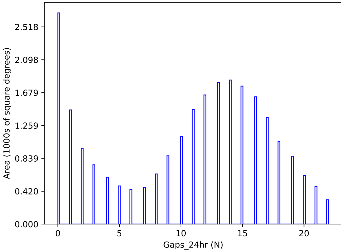
too_elab_r128_d2_ugrizy_v3.4_10yrs y band: Gaps_24hr
