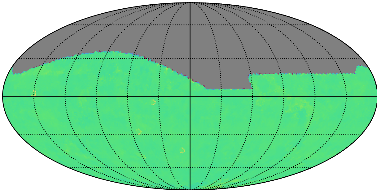
too_elab_r128_d2_gz_v3.4_10yrs i: Kuiper rotTelPos
