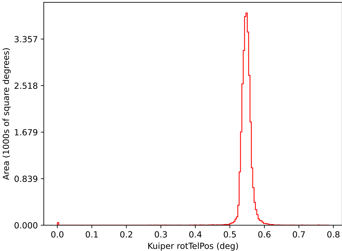
too_elab_r128_d2_gz_v3.4_10yrs i: Kuiper rotTelPos
