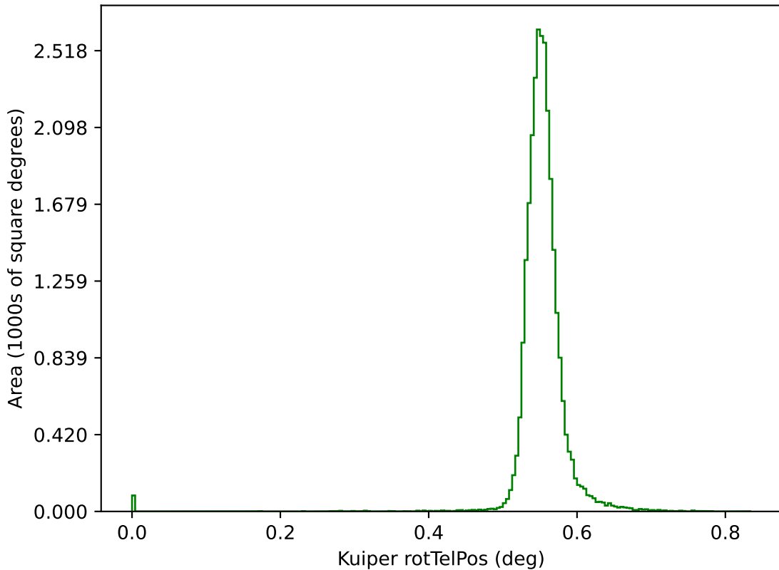
too_elab_r128_d2_gz_v3.4_10yrs g: Kuiper rotTelPos
