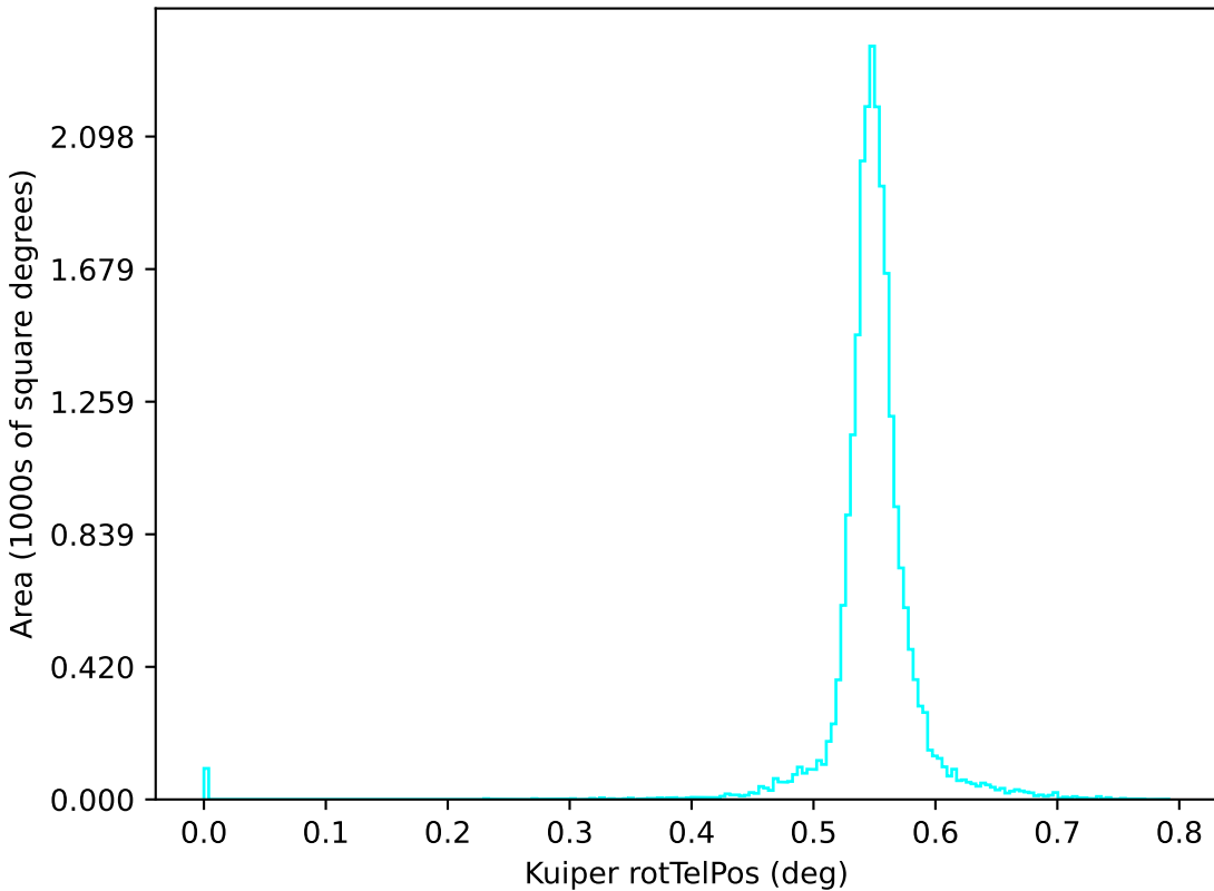
too_elab_r128_d2_griz_v3.4_10yrs u: Kuiper rotTelPos
