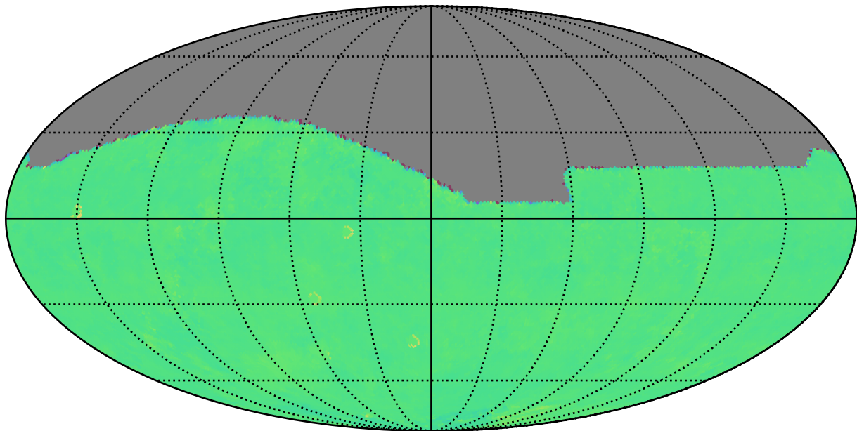
too_elab_r128_d2_griz_v3.4_10yrs i: Kuiper rotTelPos
