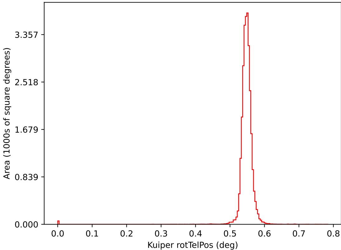
too_elab_r128_d2_griz_v3.4_10yrs i: Kuiper rotTelPos
