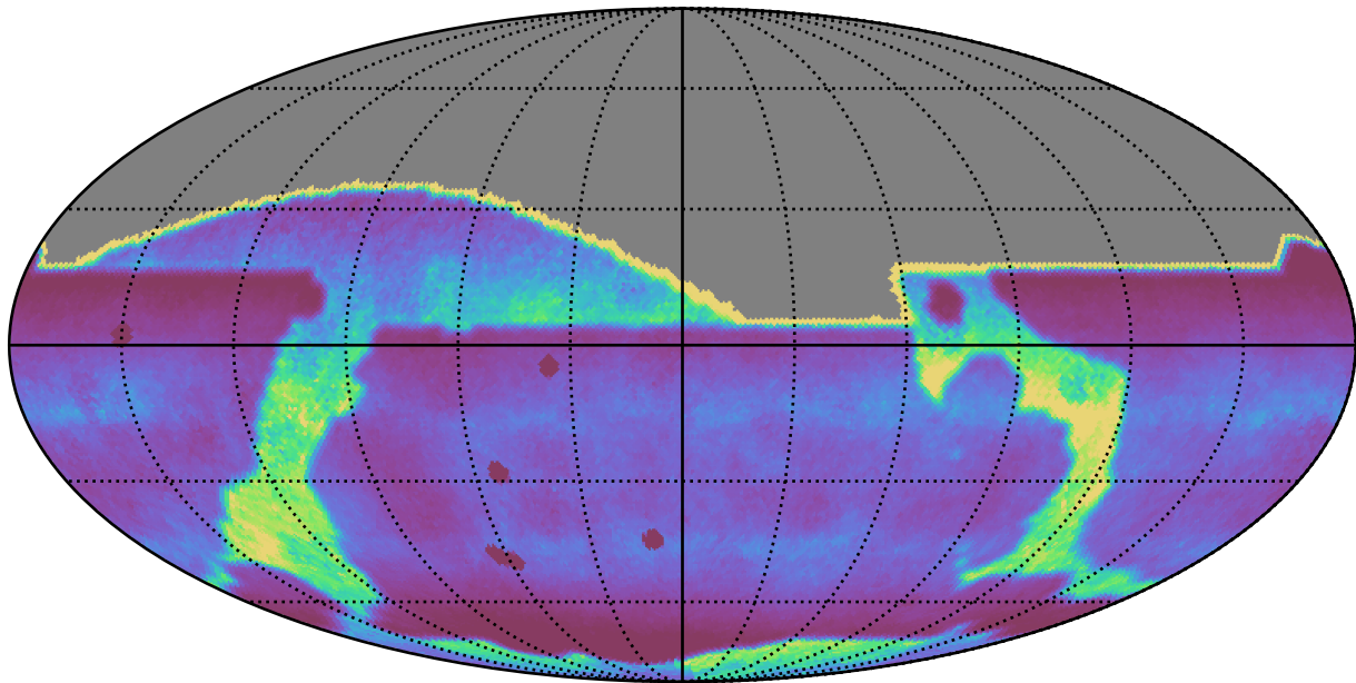
too_elab_r128_d2_griz_v3.4_10yrs : DCRprecision
