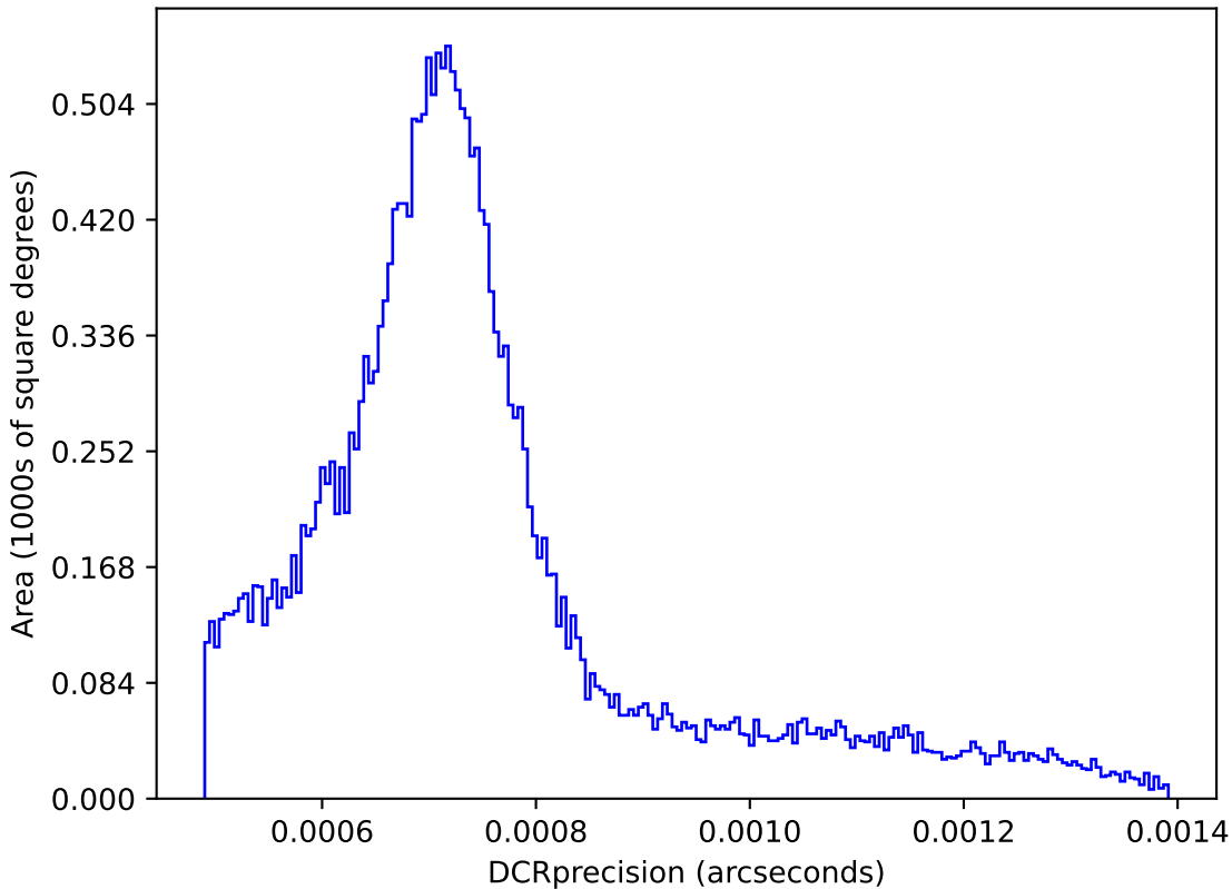
too_elab_r128_d2_griz_v3.4_10yrs : DCRprecision
