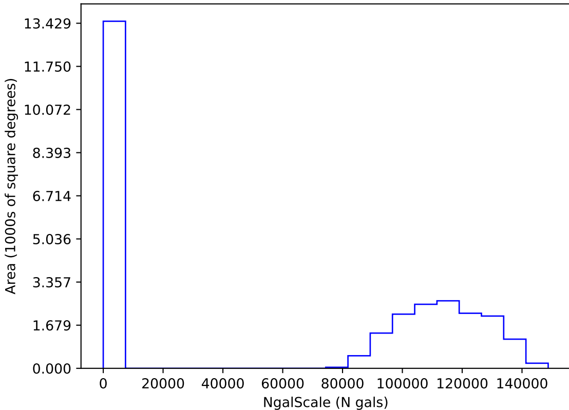
too_elab_heavy_r64_d3_ugrizy_v3.4_10yrs i: NgalScale
