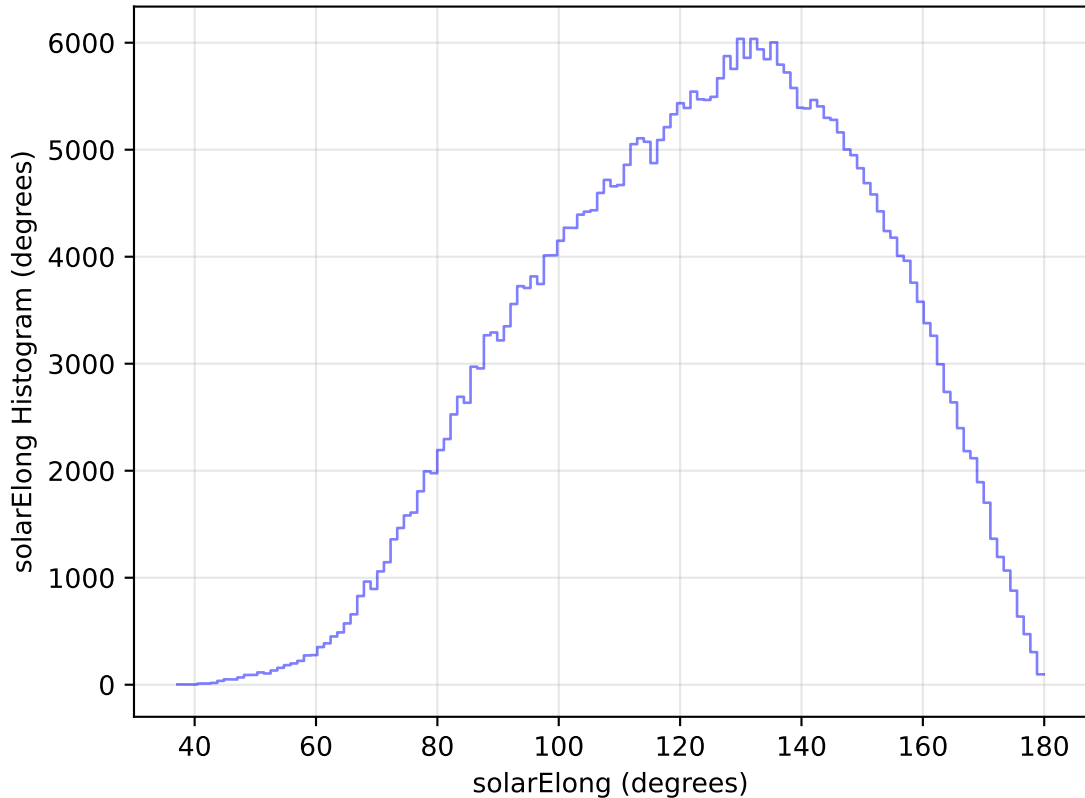
too_elab_heavy_r64_d3_ugrizy_v3.4_10yrs All sky y band: solarElong Histogram
