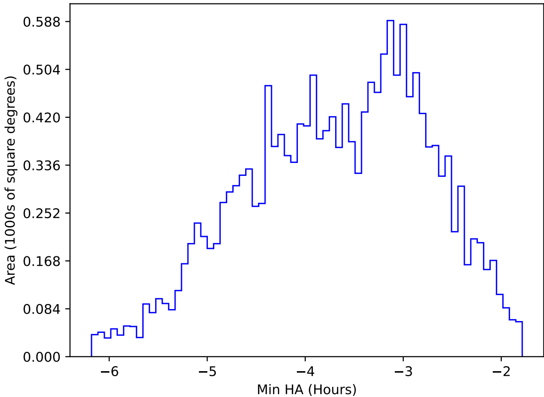
too_elab_heavy_r64_d3_ugrizy_v3.4_10yrs WFD y band: Min HA
