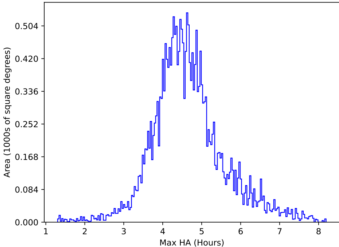
too_elab_heavy_r64_d3_ugrizy_v3.4_10yrs All sky y band: Max HA
