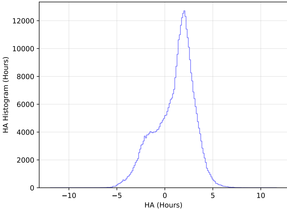
too_elab_heavy_r64_d3_ugrizy_v3.4_10yrs WFD y band: HA Histogram
