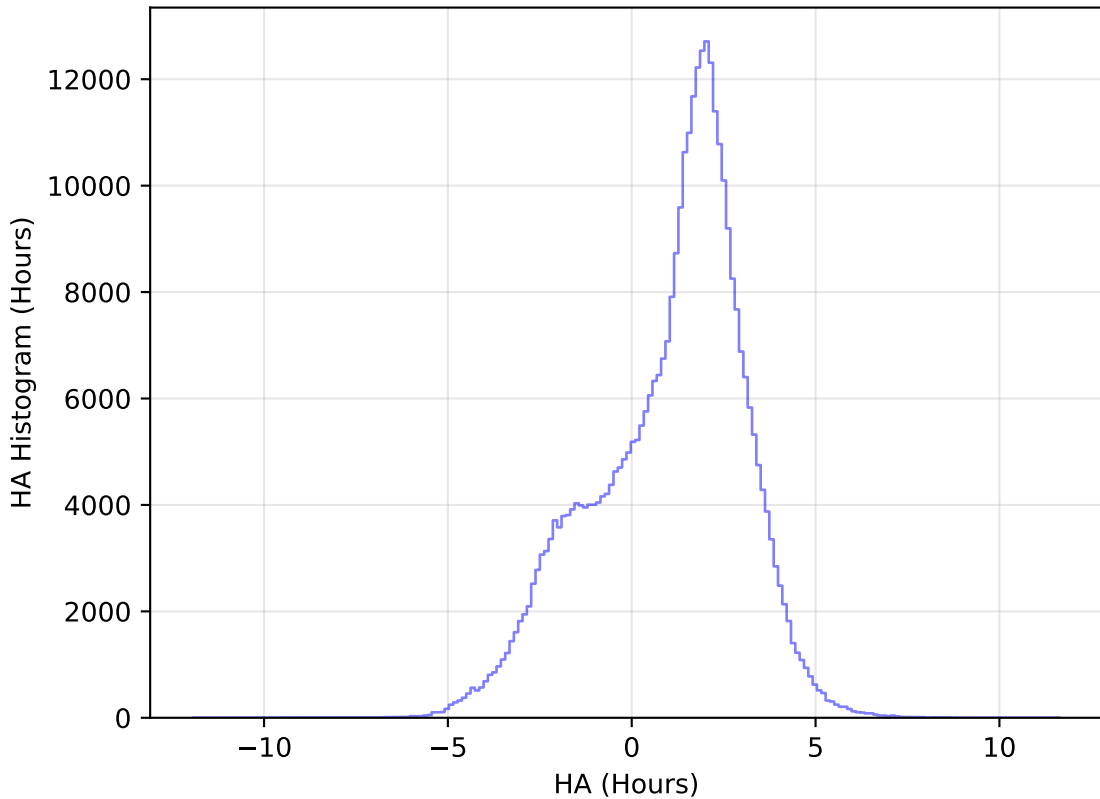
too_elab_heavy_r64_d3_ugrizy_v3.4_10yrs All sky y band: HA Histogram
