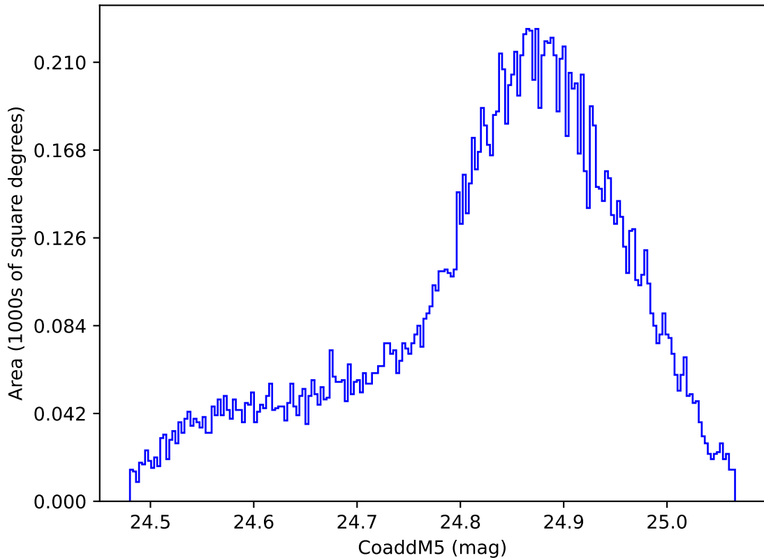
too_elab_heavy_r64_d3_ugrizy_v3.4_10yrs WFD y band: CoaddM5
