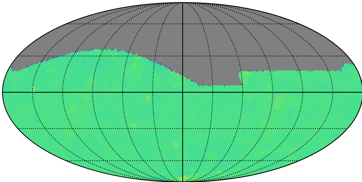
too_elab_heavy_r64_d2_ugrizy_v3.4_10yrs i: Kuiper rotTelPos
