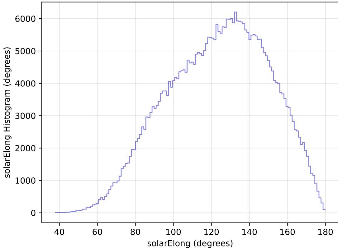
too_elab_heavy_r64_d2_ugrizy_v3.4_10yrs All sky y band: solarElong Histogram
