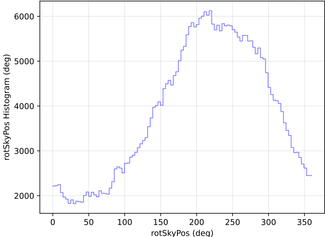
too_elab_heavy_r64_d2_ugrizy_v3.4_10yrs All sky y band: rotSkyPos Histogram
